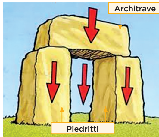
Schema sistema trilitico (cioè con tre pietre).
